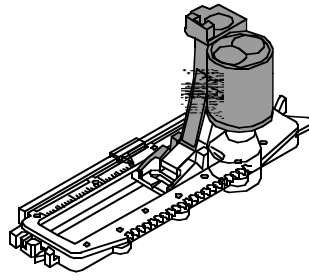
3A Knopflochschlittenfuss Knopflöcher in flachen Materialien, Stopfprogramme
